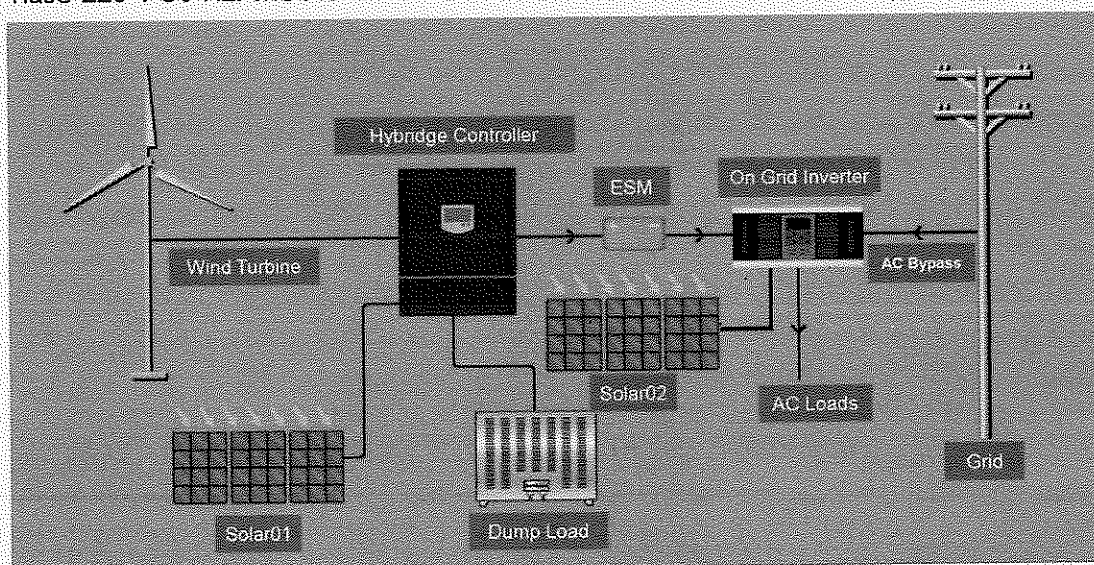
รูปที่ 1 ระบบผลิตไฟฟ้าพลังงานร่วมระหว่างพลังงานลมและพลังงานแสงอาทิตย์ชนิด Hybrid
